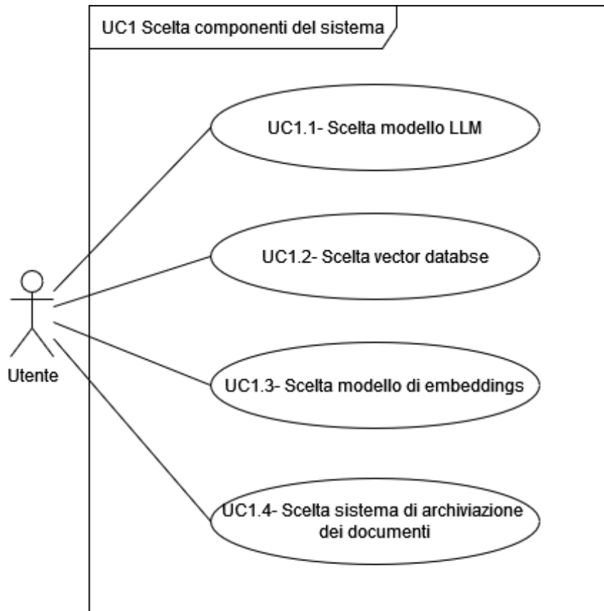
Figura 5: Diagramma UC1
